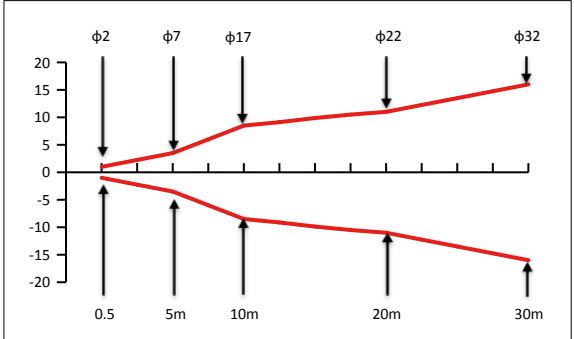
OSQ18-SL 光斑图 单位 (mm)
