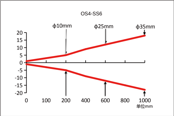
OS4-SS6 光斑图 单位 (mm)
