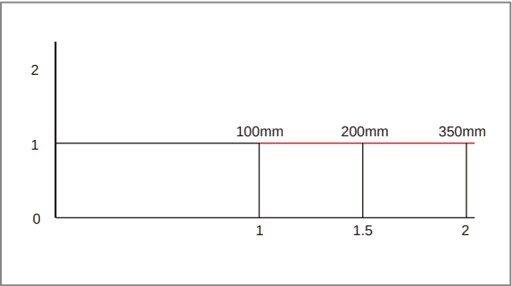
OS10-AKL(AKL150|AKL350) 光斑图 (mm)
