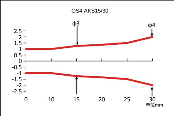
OS4-AKS15/30 光斑图 单位 (mm)
