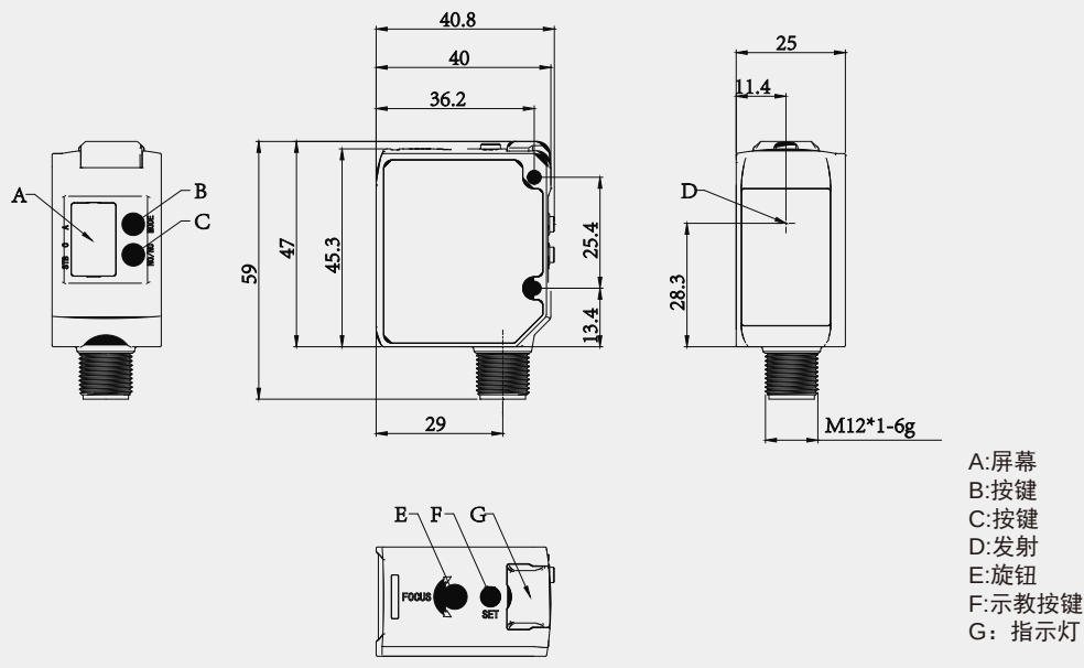
M12接插件
